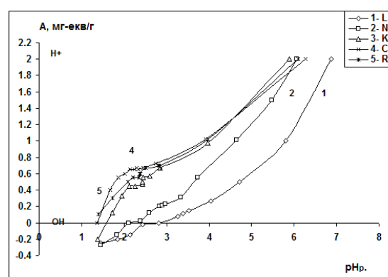
Рис. 5. Криві рН-метричного титрування ТС(Н-форма) 0,1N HCl та MOH на тлі 0,1N MCl, де М – Li, Na, K, Rb, Cs
